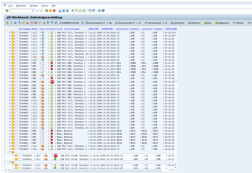
Abbildung 1 QS-Workbench
